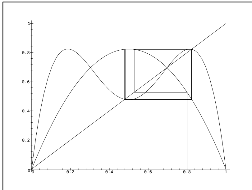
Fig. 4. x_0 = 0.8 en a = 3.3 , de nieuwe grafiek is die van f_2
