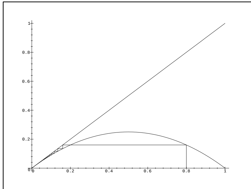
Fig. 7. a = 1 .
